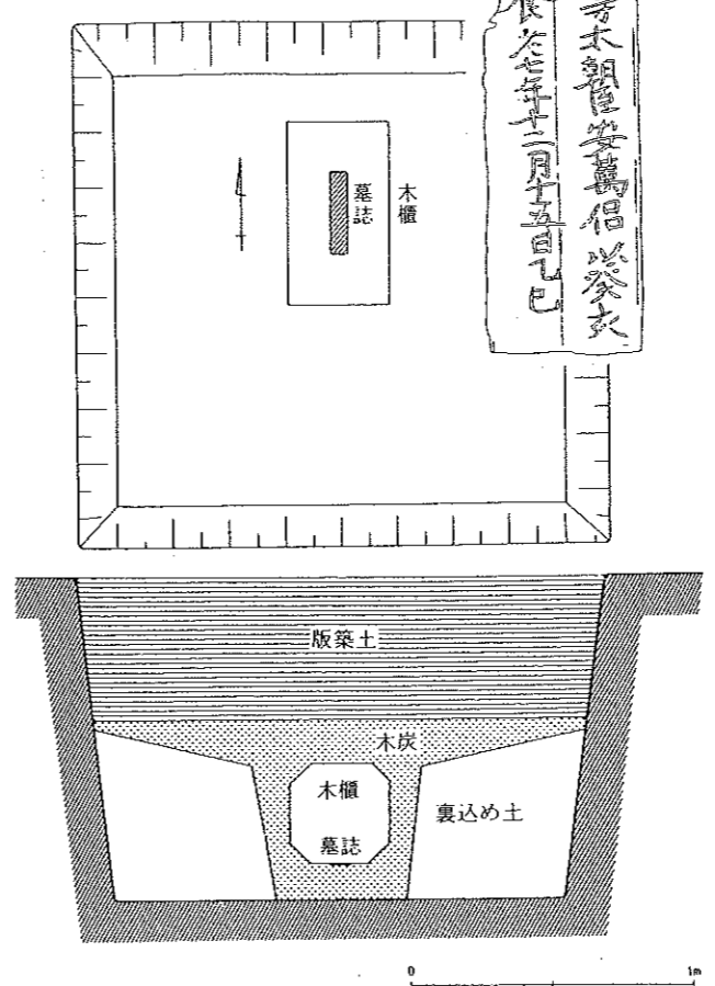
遺構模式図(上・平面図, 下・断面図)
