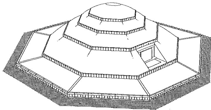
天武・持統陵墳丘復元図
