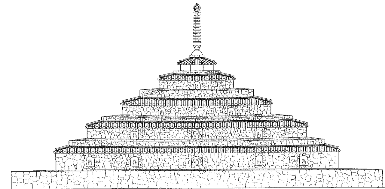
復原立面図
