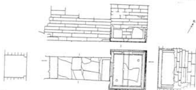
图一七六 石表
