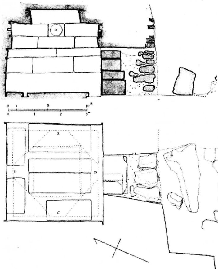
通溝四神塚墓室平立面圖
