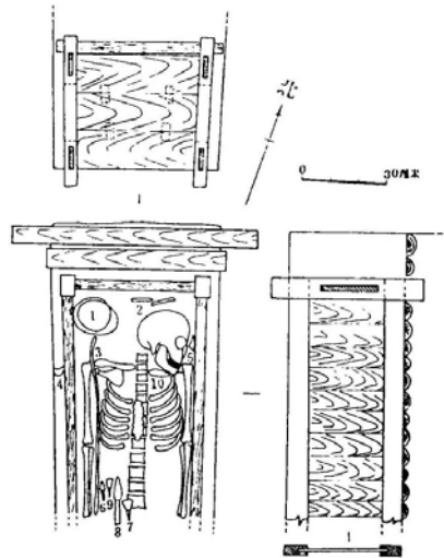
图二 M2 平剖面图
