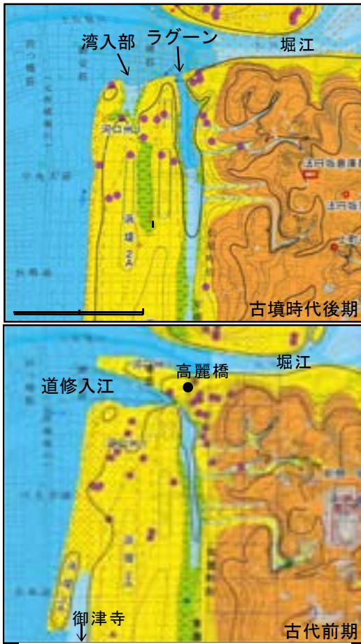
図1 上町台地の古地形と難波津の推定 (古地理図は[趙・中条 2017])
