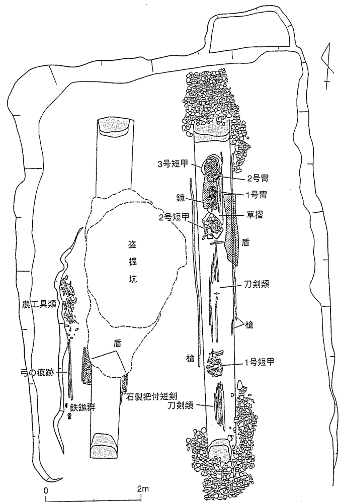
大阪府 大塚古墳第2主体部(右東榔、左西榔)
